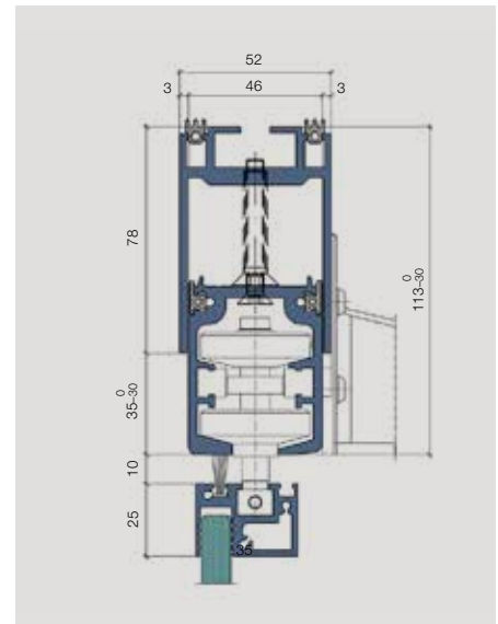
Detail oben mit Ausgleichsprofil 78 mm Profile auf Maximalmass +20 mm
