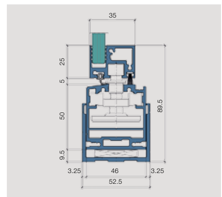
Detail unten mit Ausgleichsprofil
