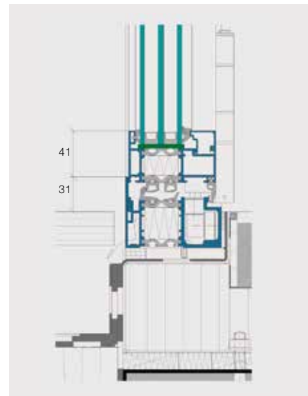
Coupe verticale, partie basse, ouvrant vers l'intérieur
