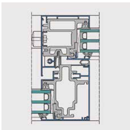
Horizontalschnitt Mittelpartie
