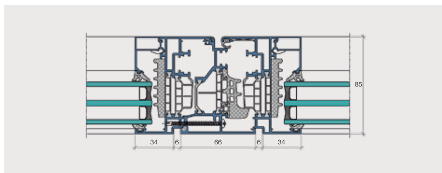
Coupe horizontale fenetre IS-4 partie centrale (côte)
