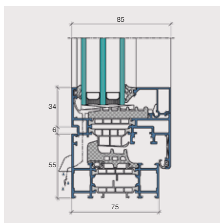
Coupe verticale fenetre IS-4
