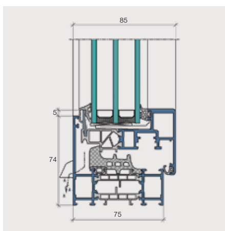
Coupe verticale fenetre IS-4 à ouvrant caché
