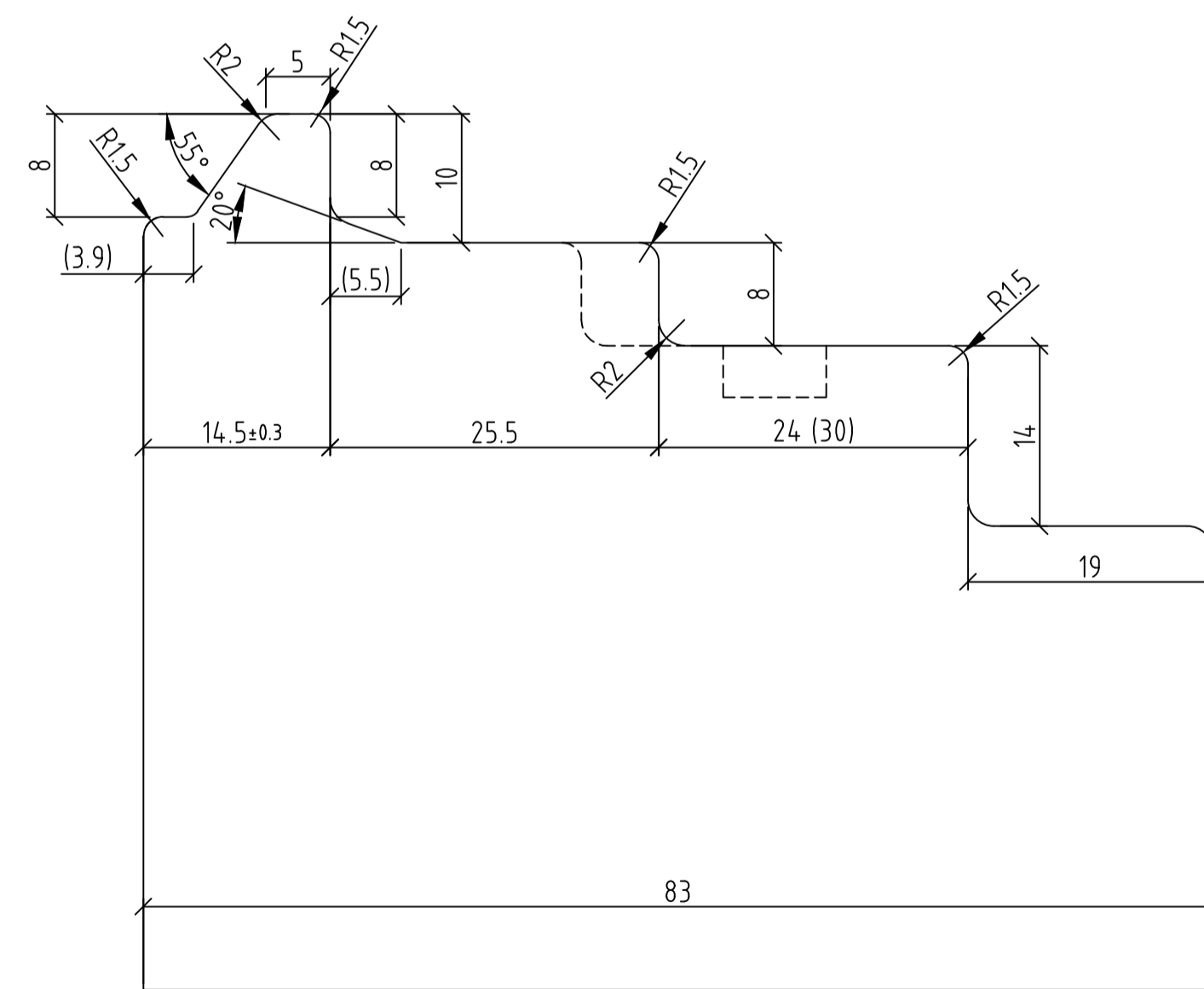
Rahmenfälzung 4-seitig
