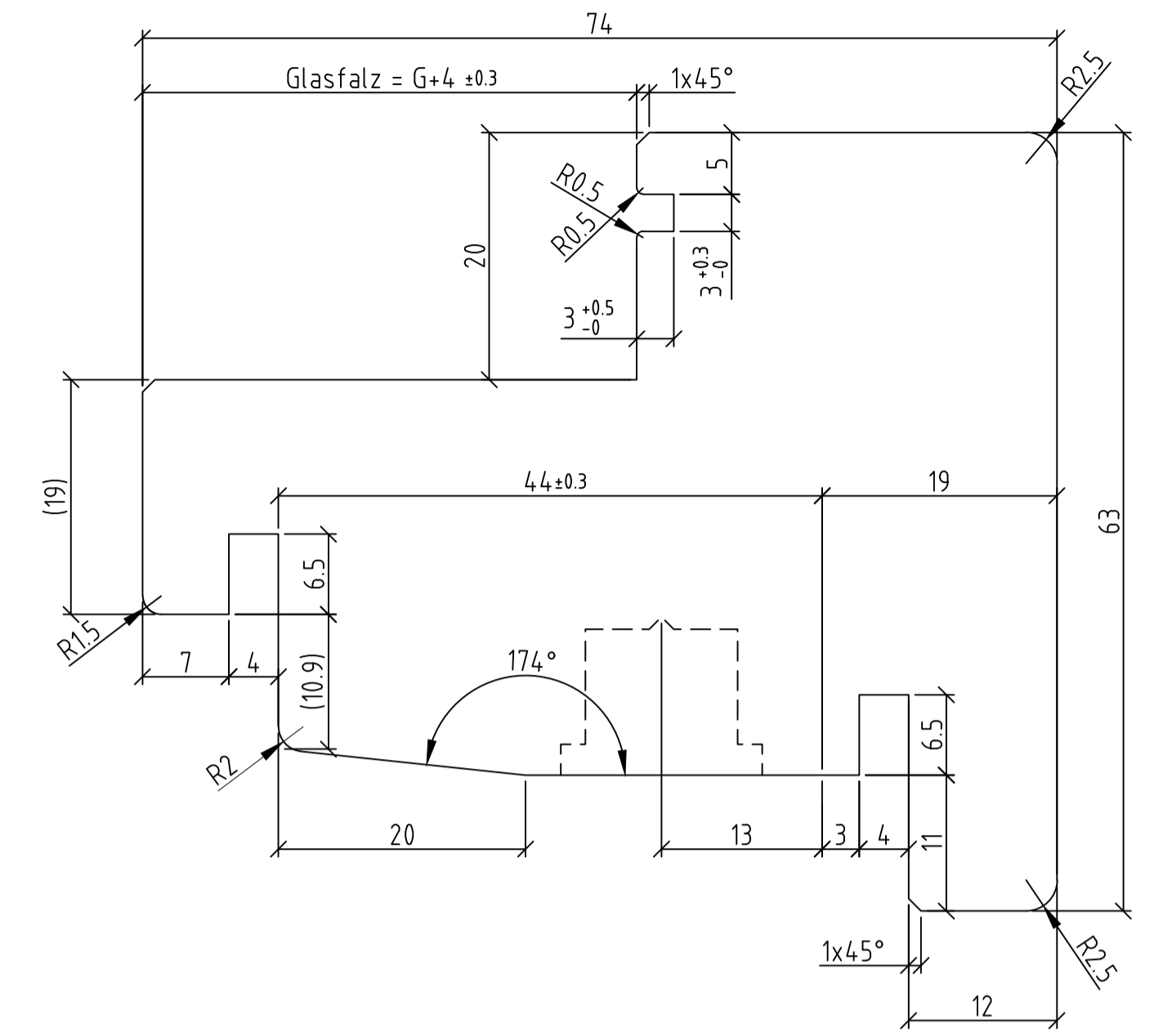
rollstuhlg. Schwelle
