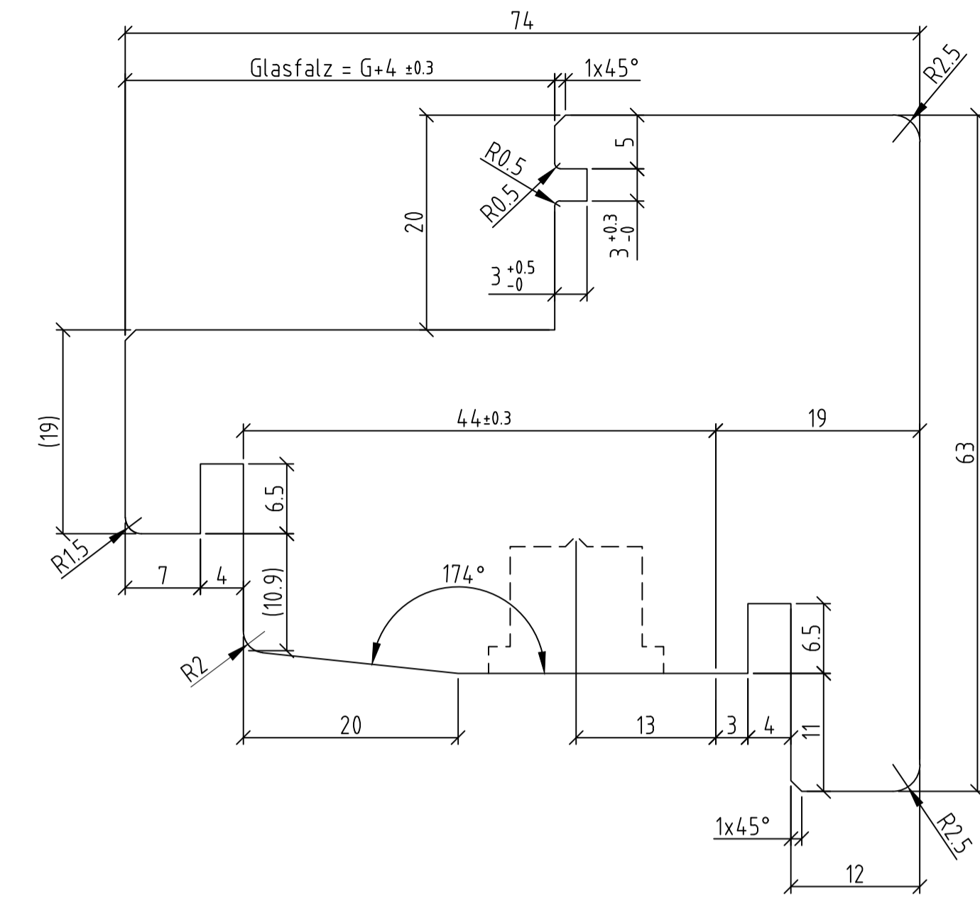
rollstuhl. Schwelle
