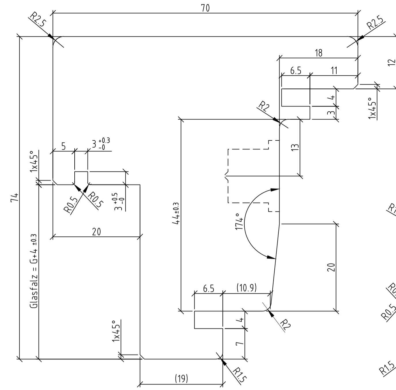
Flügelfälzung
