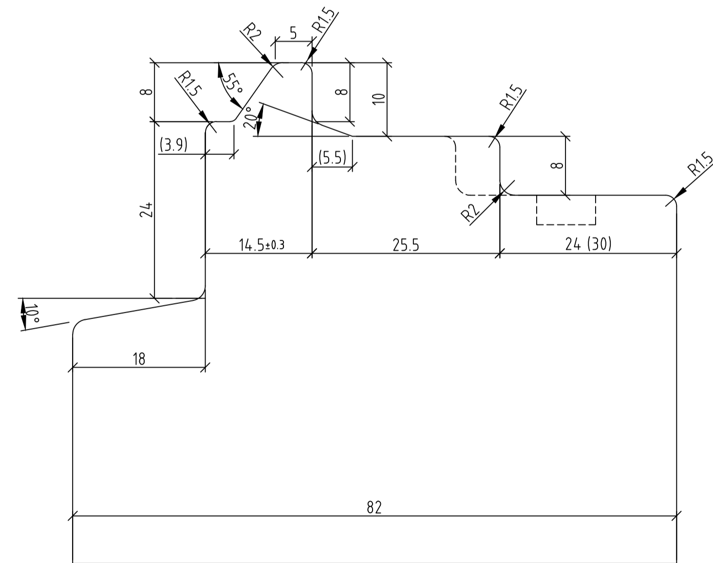
Rahmenfälzung 4-seitig
