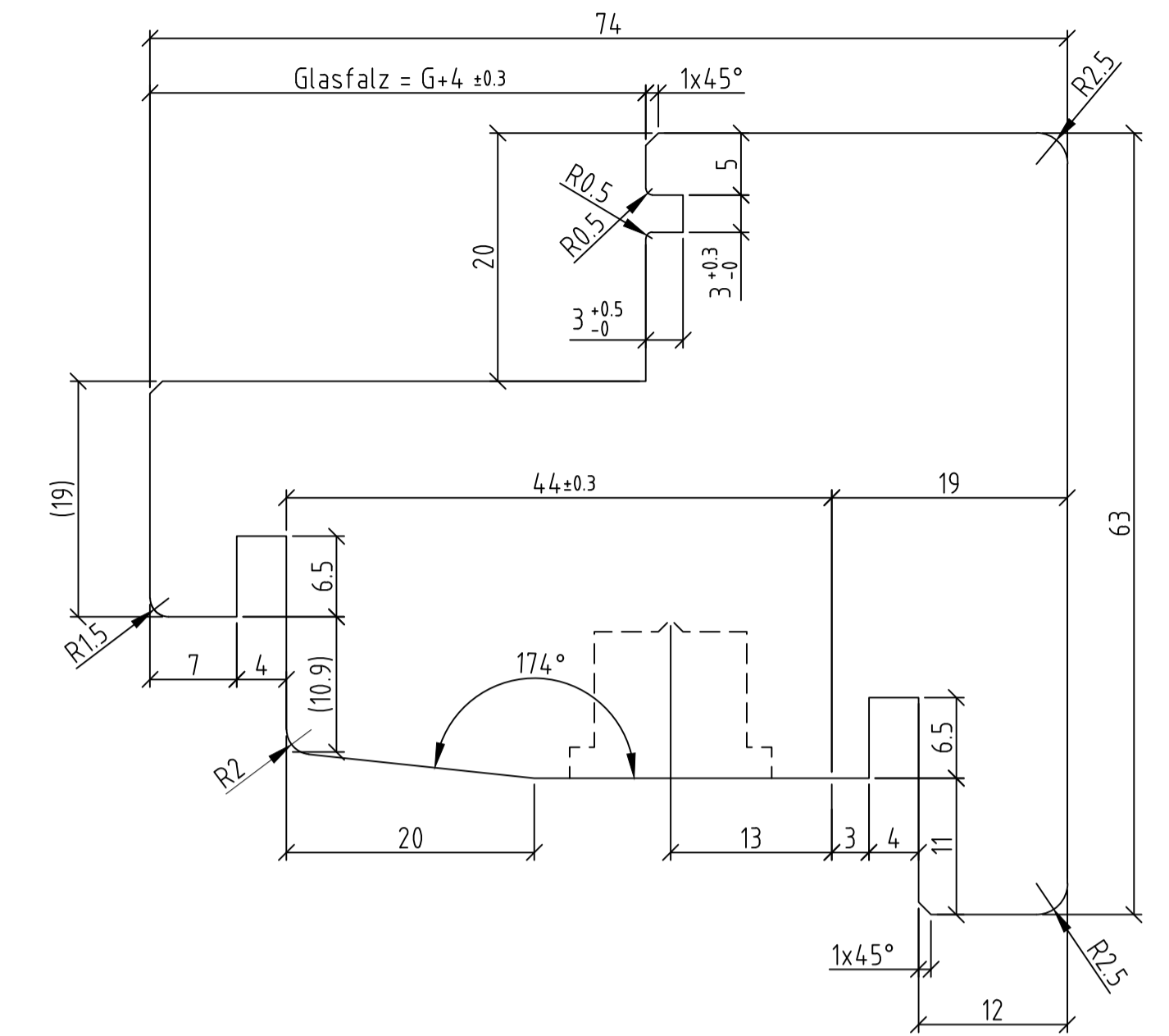
rollstuhlg. Schwelle
