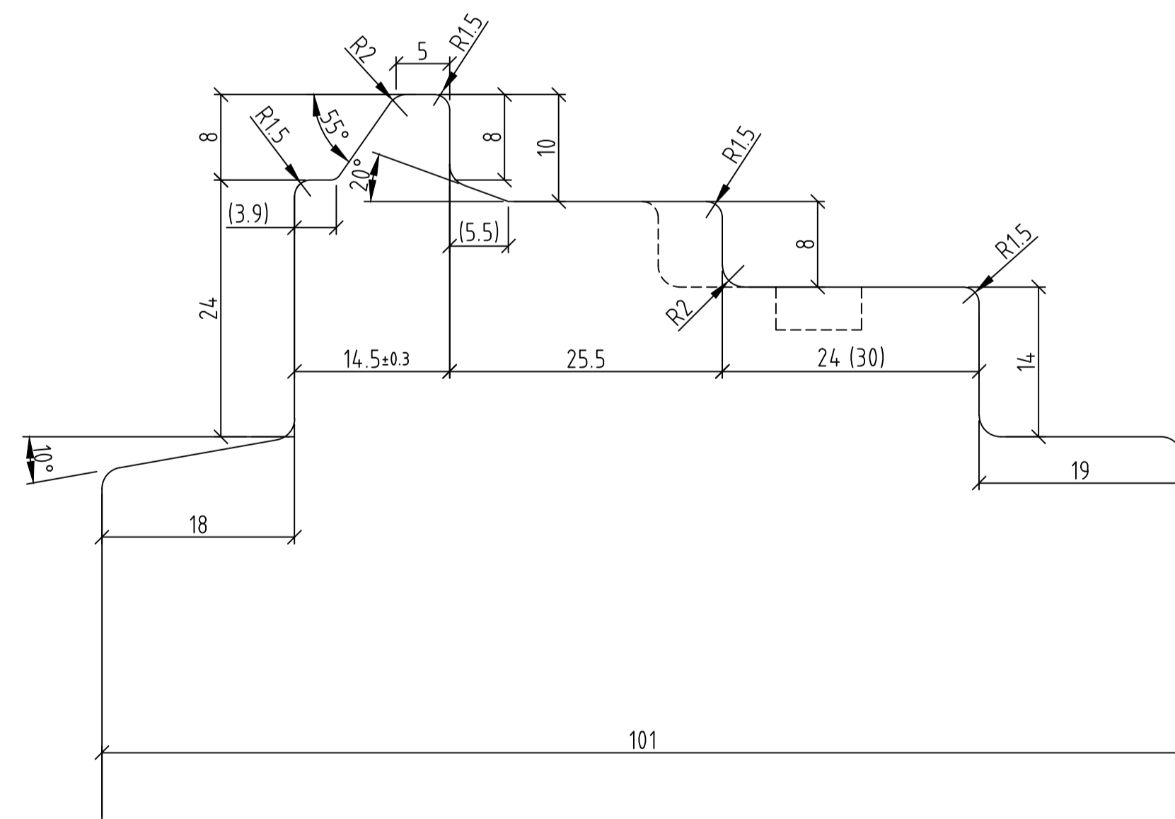
Rahmenfälzung 4-seitig
