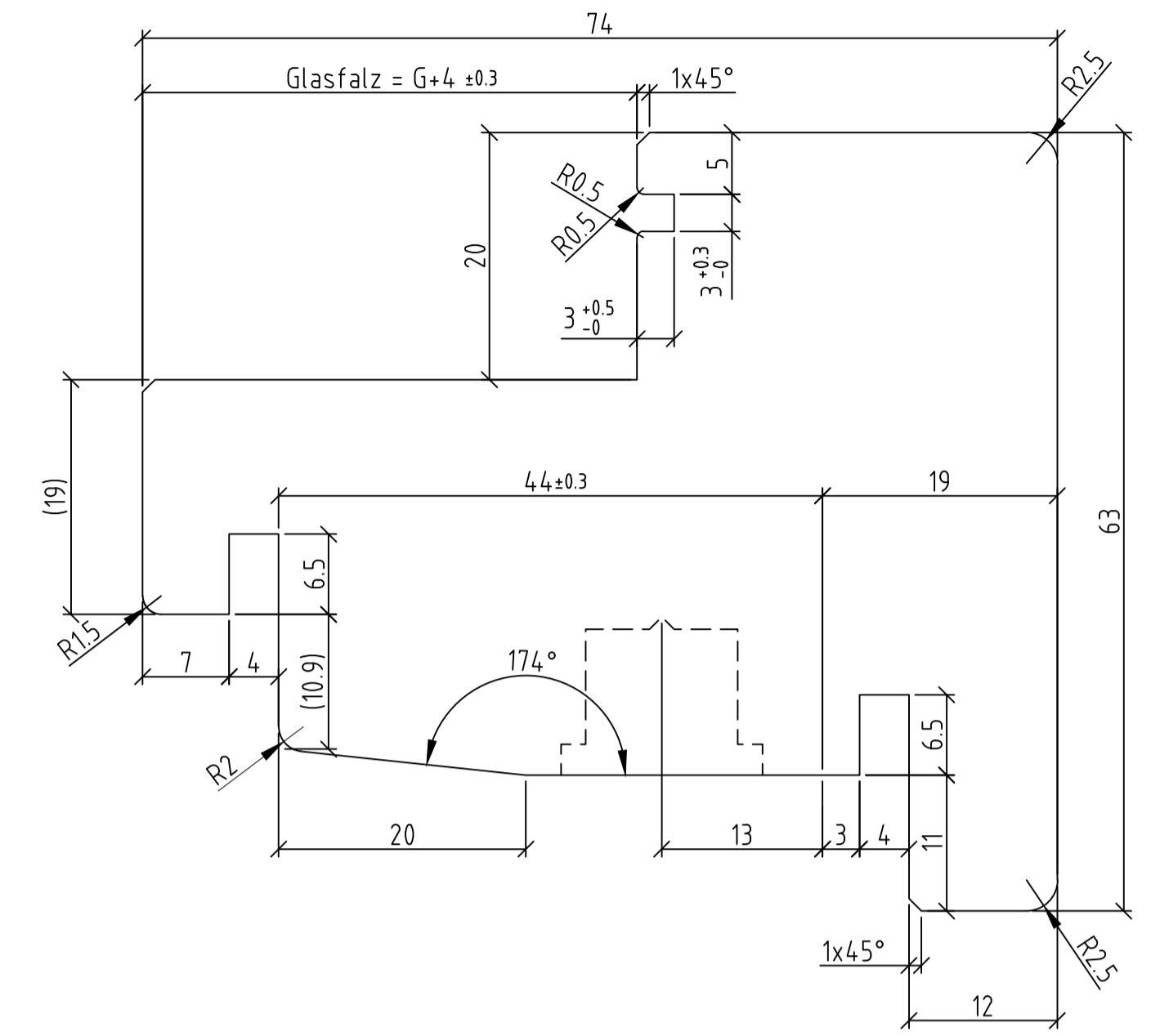
rollstuhlg. Schwelle
