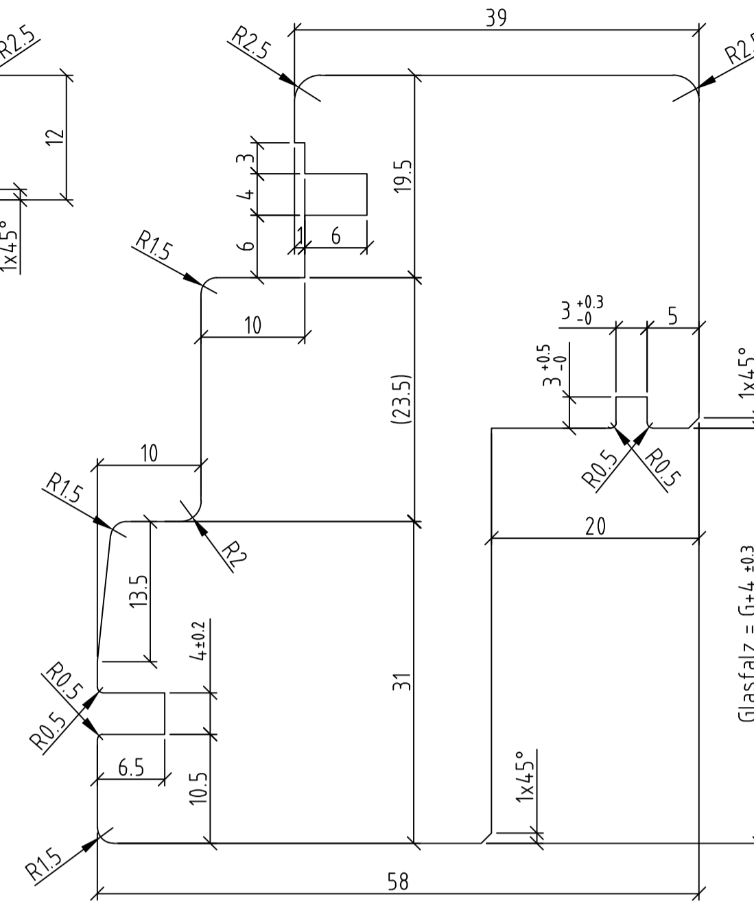
Stulp
