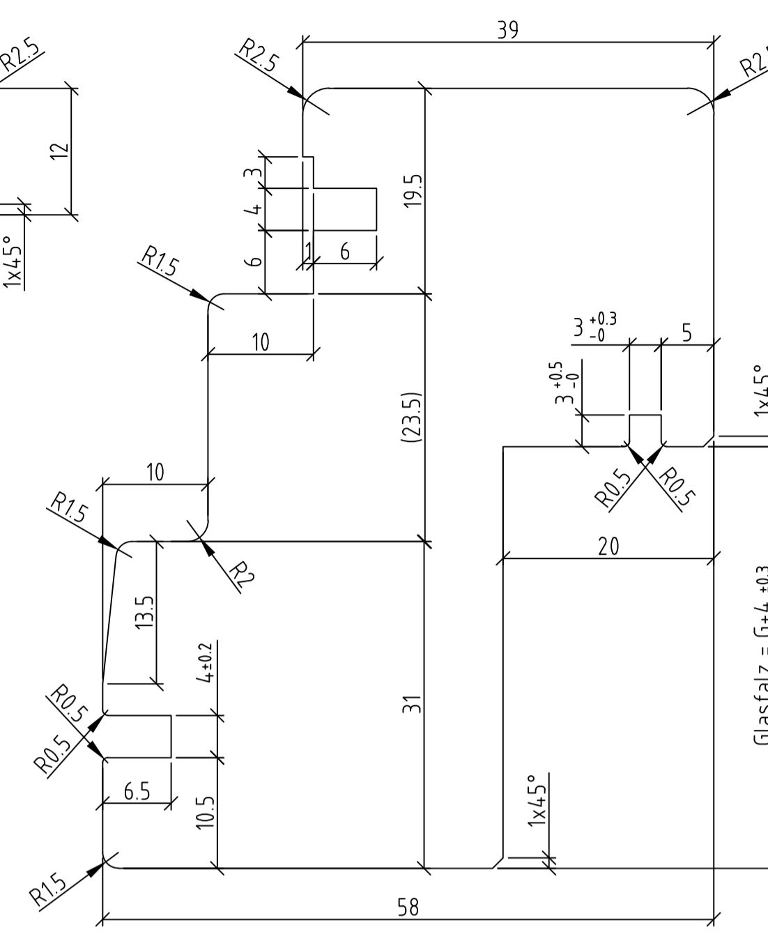
Stulp
