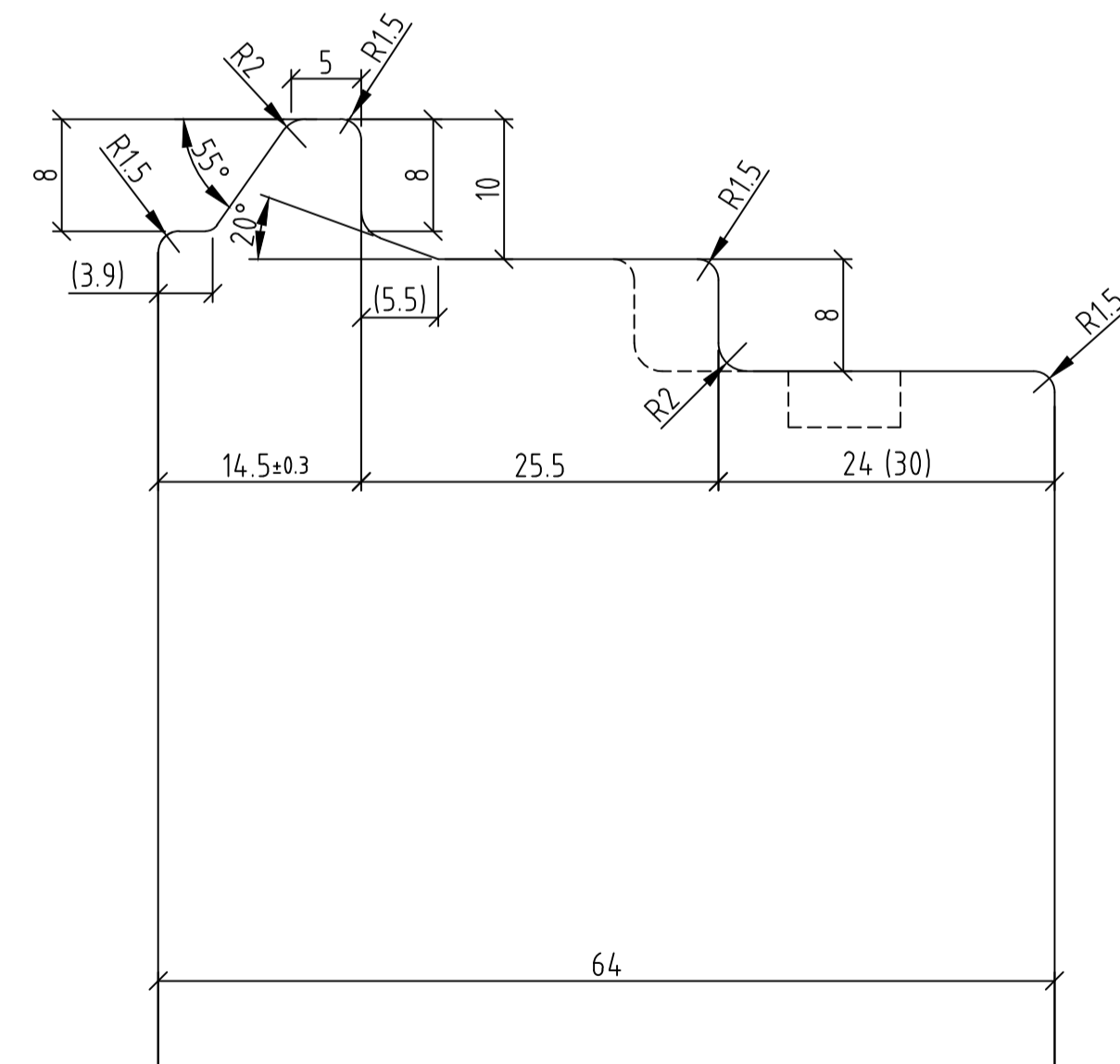
Rahmenfälzung 4-seitig
