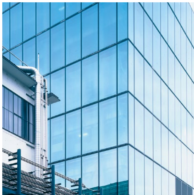
Construction de base en acier, vitres collées sur des cadres en aluminium selon la technique SSG Bâtiment de production Roche 95, Bâle
