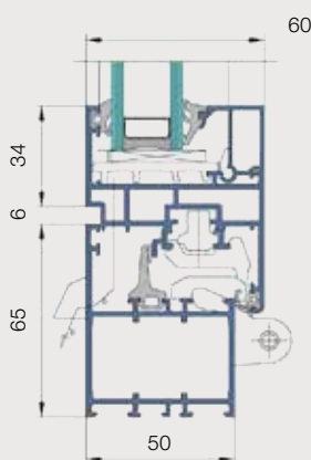
Fenêtre aldura basic: coupe verticale
