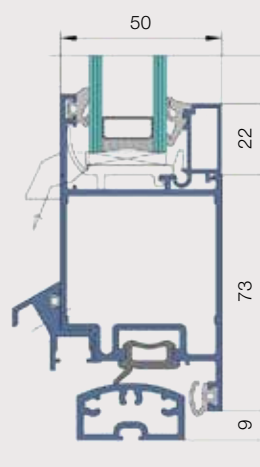
Porte aldura basic: coupe verticale avec ouverture vers l'intérieur
