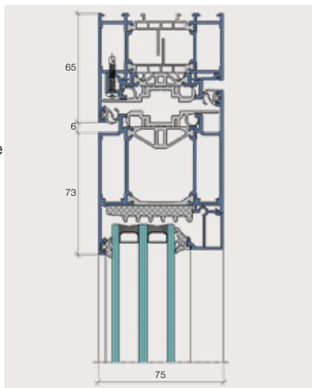
Coupe verticale de la porte aldura comfort, partie supérieure, ouverture vers l'intérieur
