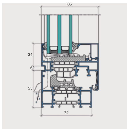
Coupe verticale fenetre aldura comfort
