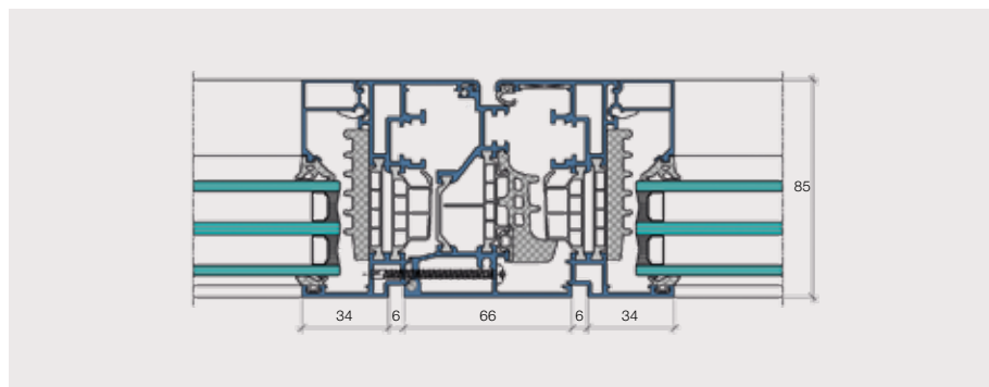
Coupe horizontale fenetre aldura comfort partie centrale (côte)
