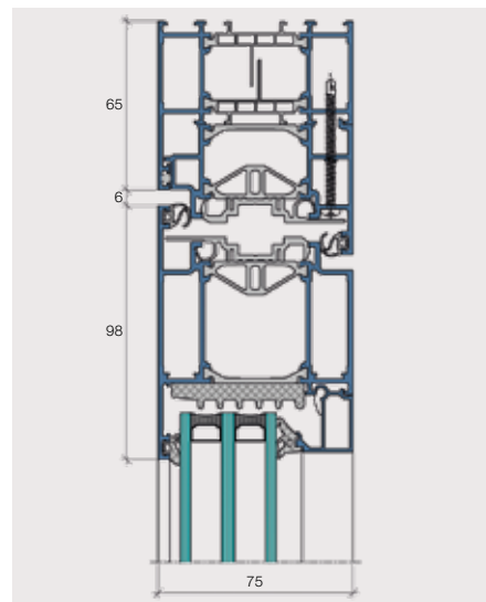
Coupe verticale de la porte aldura comfort, partie supérieure, ouverture vers l'extérieur
