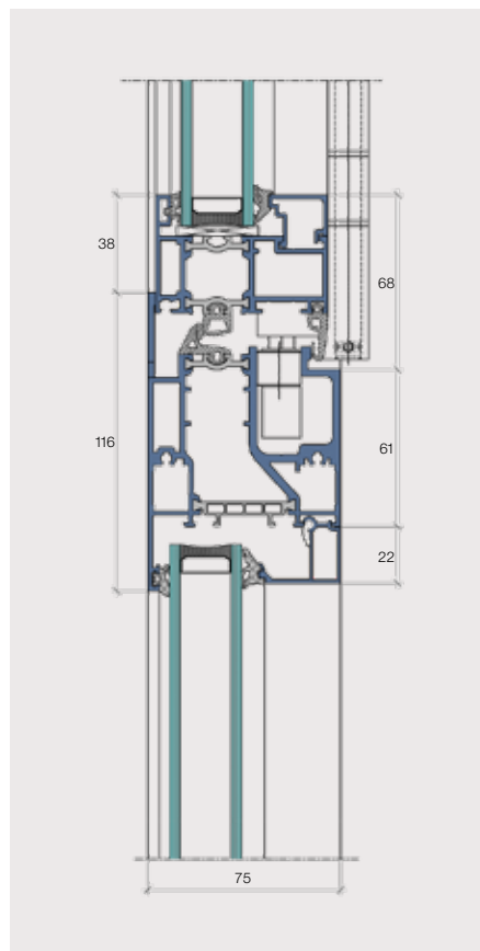
Coupe verticale durafold comfort sur allège aldura comfort
