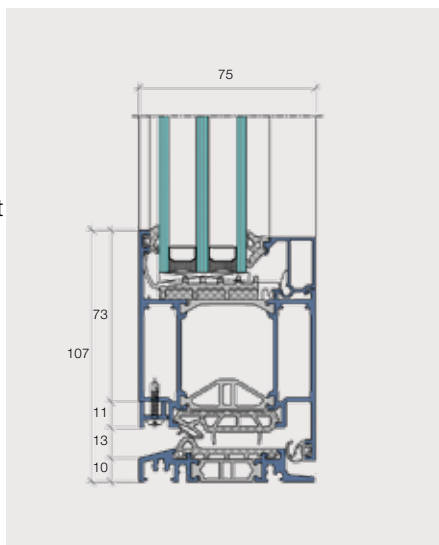
Coupe verticale de la porte aldura comfort, partie inférieure, ouverture vers l'intérieur
