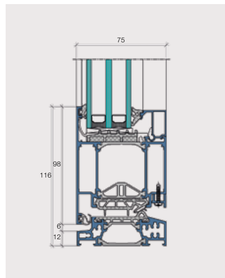
Coupe verticale de la porte aldura comfort, partie inférieure, ouverture vers l'extérieur
