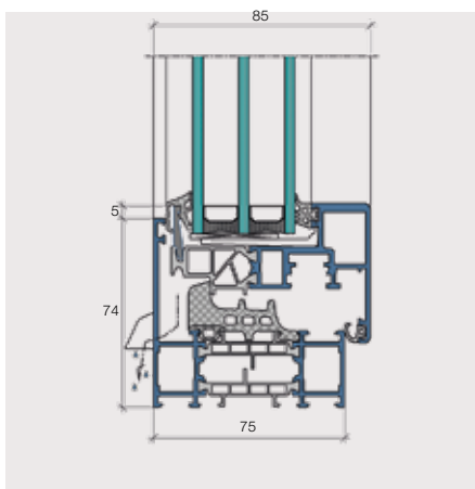
Coupe verticale fenetre aldura comfort à ouvrant caché
