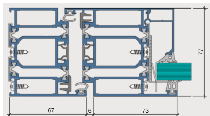
Coupe horizontale aldura fuego EI30/T30
