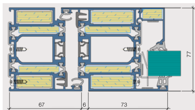
Coupe horizontale aldura fuegoS EI60/T60
