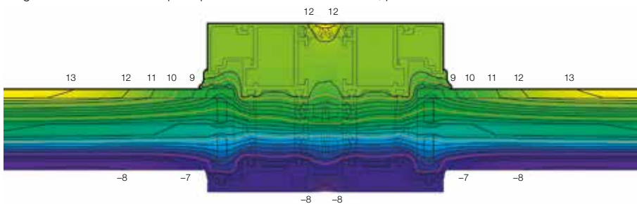
Diagramme isotherme de la paroi pliante vitrée durafold comfort+, partie médiane
