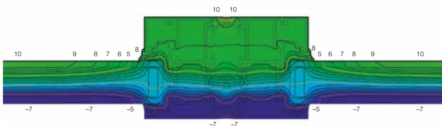
Diagramme isotherme de la paroi pliante vitrée durafold comfort, partie médiane
