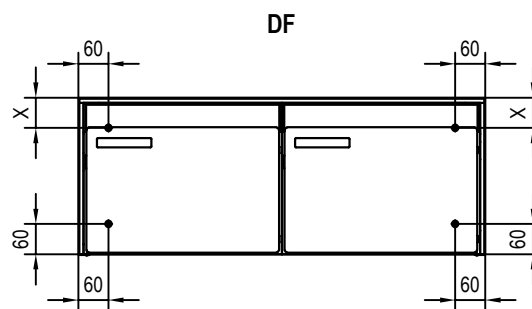
Exécution DF fixée avec 4 vis
